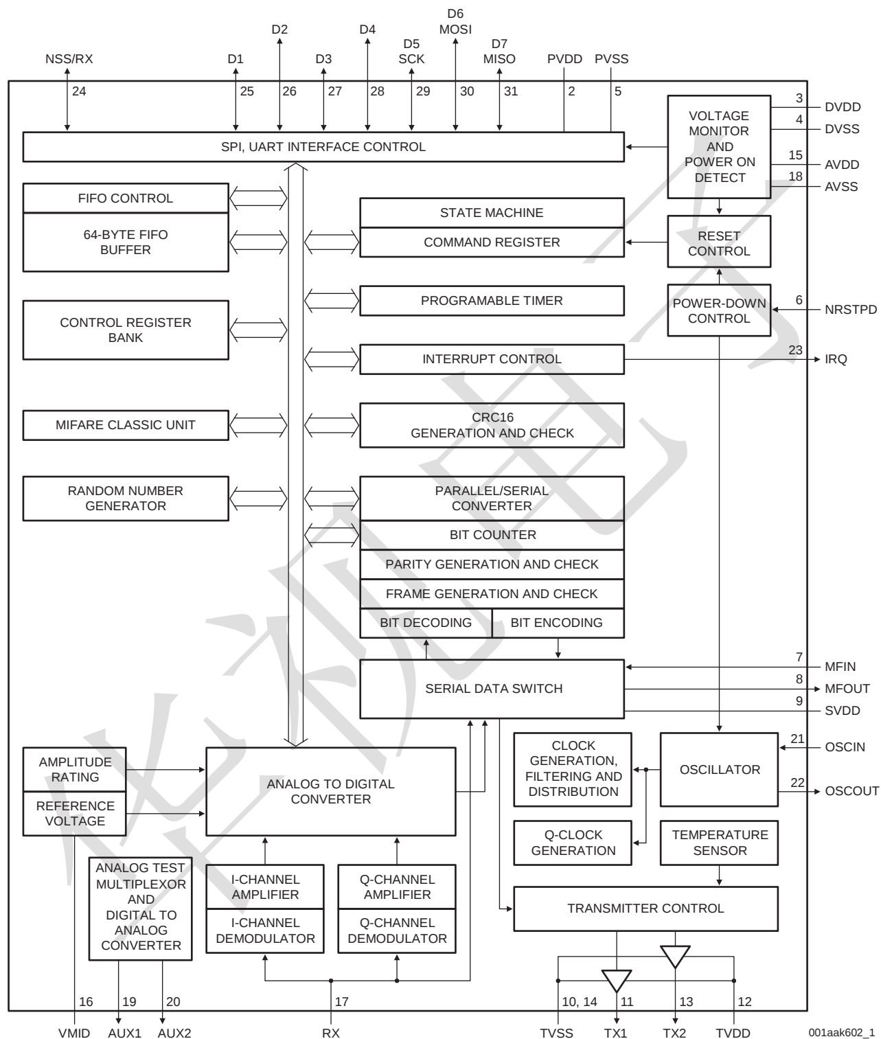
Fig 2. MF CV520 详图
