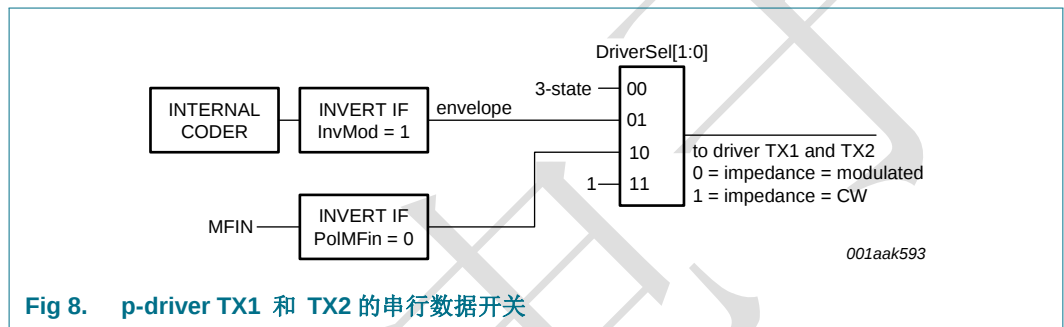
Figure 8 p-driver 的 TX1 和 TX2 的串行数据开关
